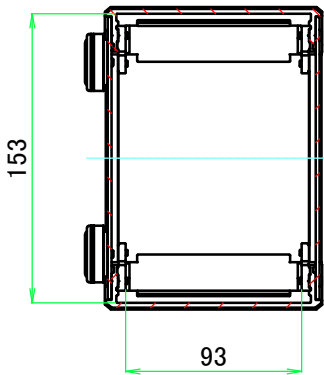
B-B ( 1 : 4 )
