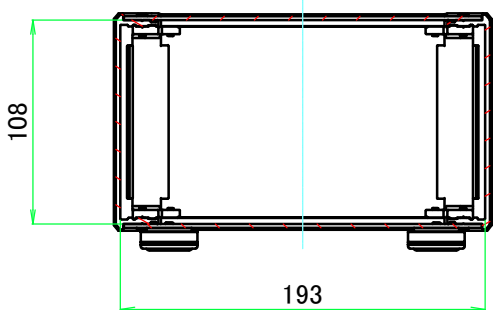
A-A ( 1 : 4 )
